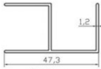
K4411 DİKME BAĞLANTI (0.395 Kg/m)
