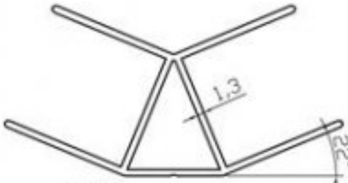
K4410 KÖŞE PROFİLİ (135°) (0.570 Kg/m)
